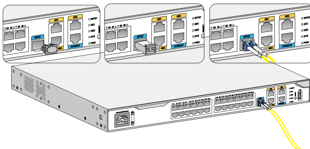
图2-15 连接以太网光口线缆
