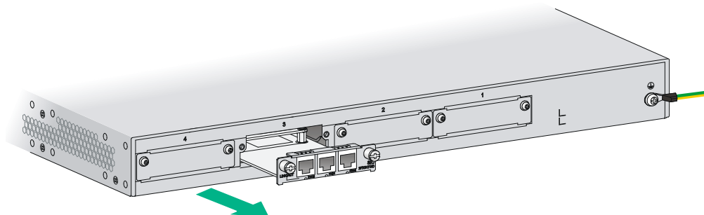
图3-4 拆卸 SIC 接口模块
