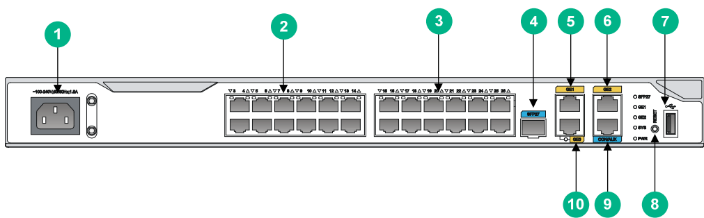
图A-1 R3900-S28 前视图
