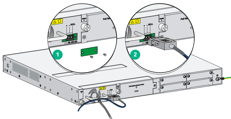
图2-20 R3600-51 设备连接直流电源线
