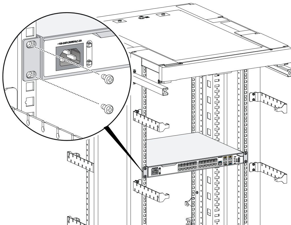
图2-10 安装设备到机架
