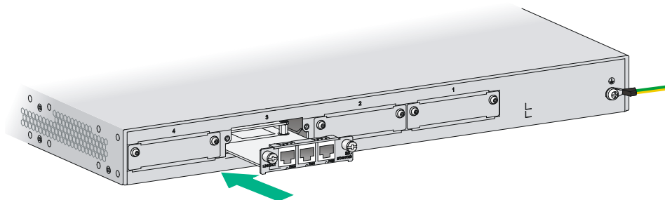
图2-13 安装 SIC 接口模块
