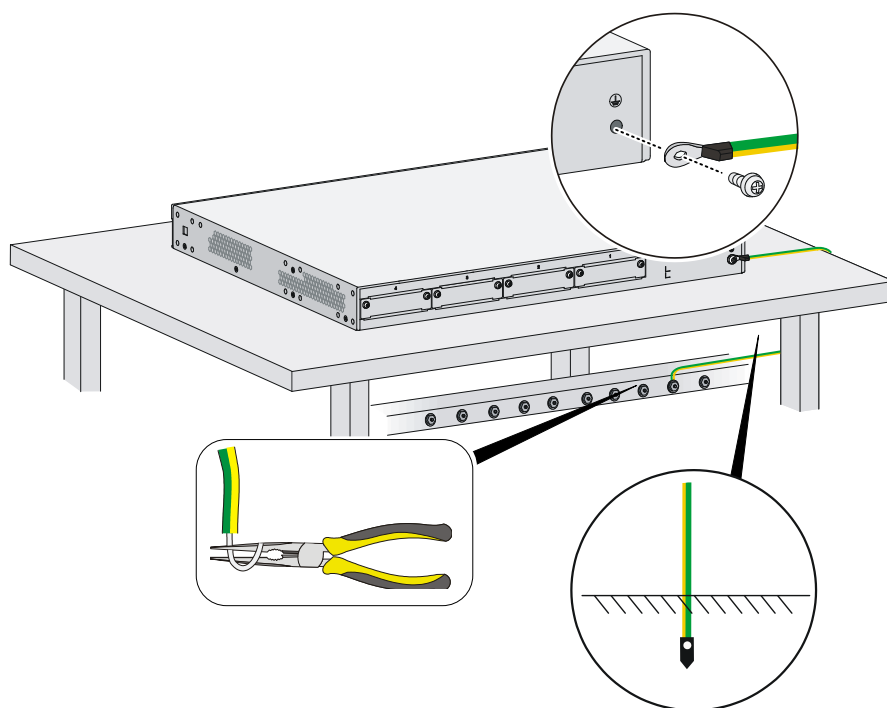
图2-12 通过接地排接地.
