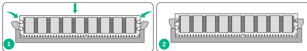
图3-3 安装内存
