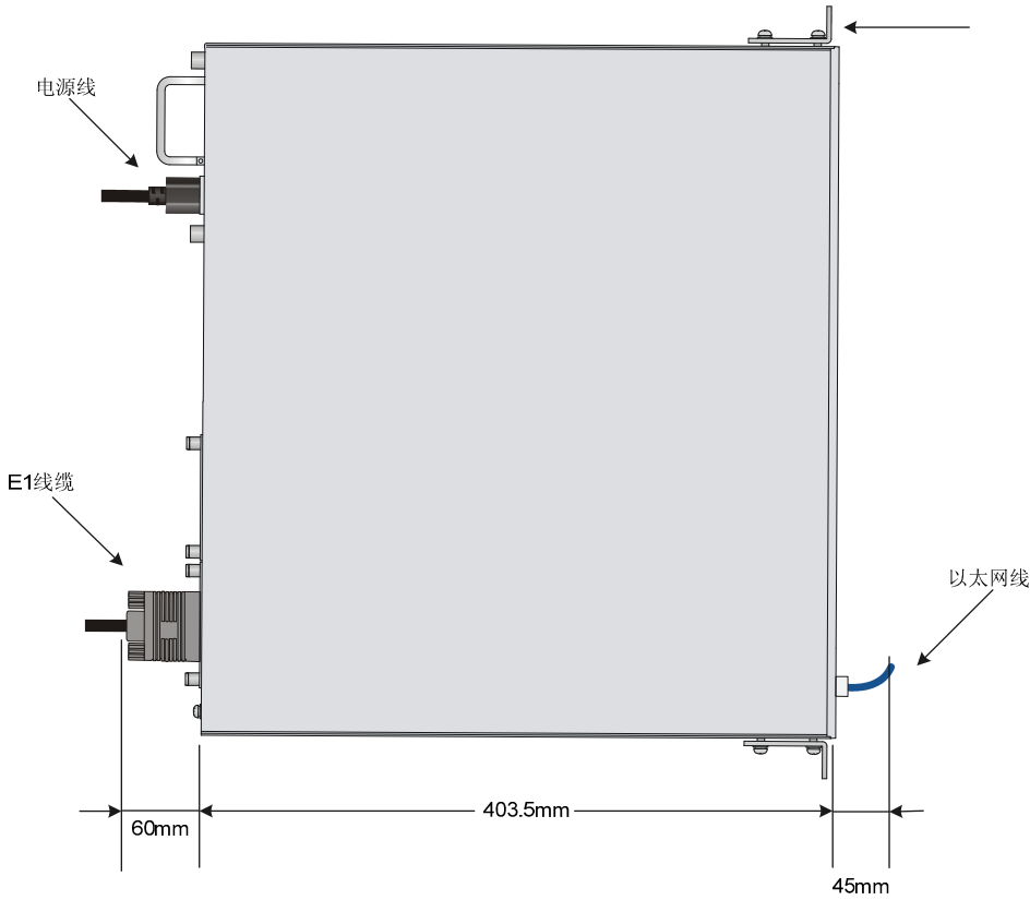
图2-6 R3900-S51 设备尺寸
