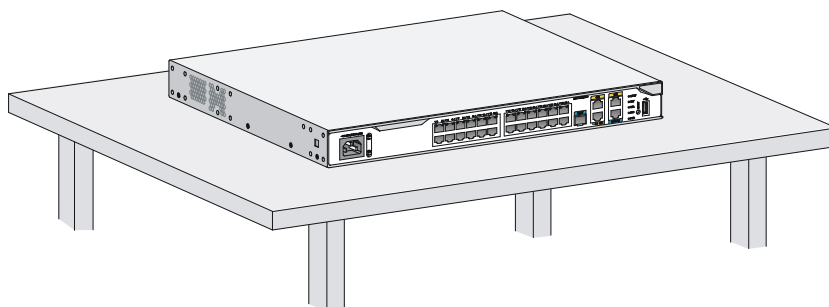
图2-3 安装设备到桌面
