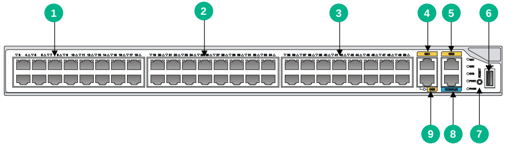
图A-3 R3900-S51 前视图
