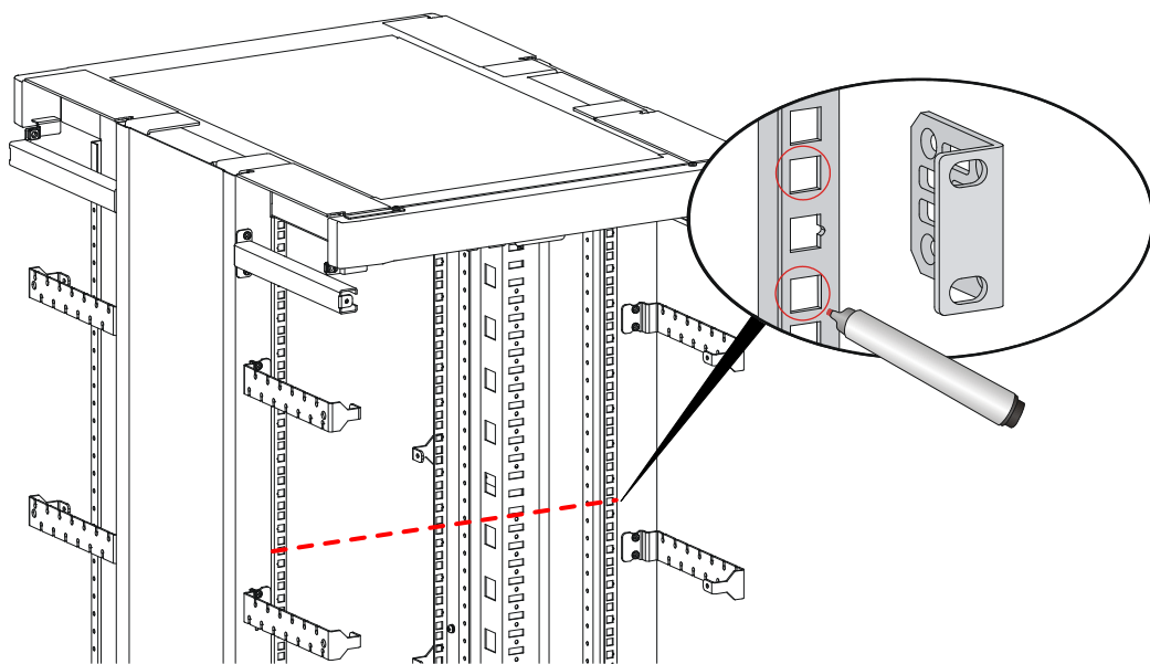
图2-7 标记挂耳浮动螺母安装位置
