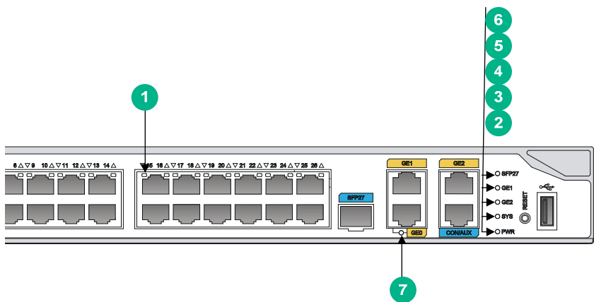
图B-1 R3900-S28 指示灯
