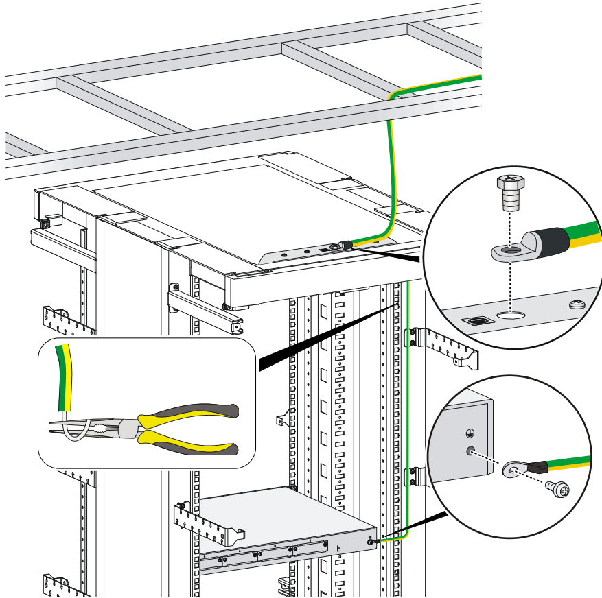
图2-11 机架方式安装接地线
