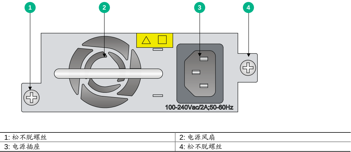
图A-5 R3900-S51 交流电源模块
