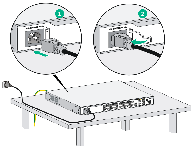
图2-19 设备连接交流电源线
