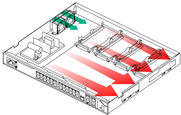
图1-1 R3900-S28/R3900-S51 的散热方式
