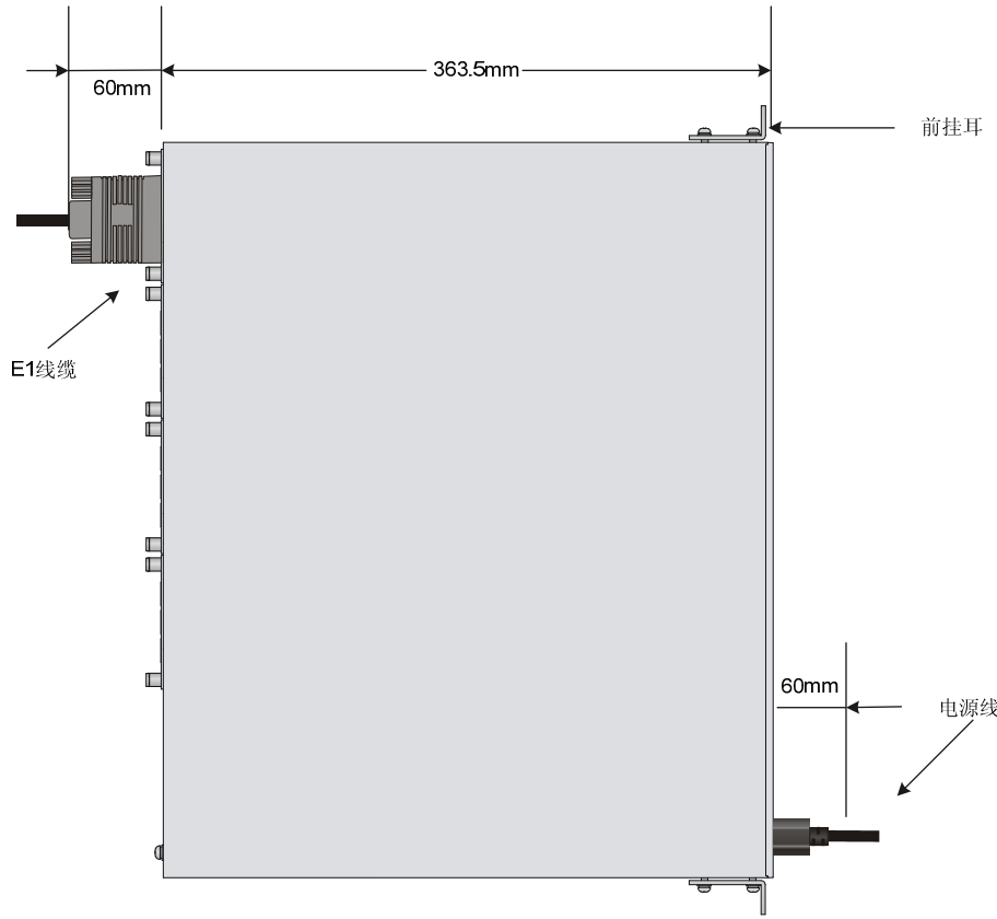
图2-5 R3900-S28 设备尺寸
