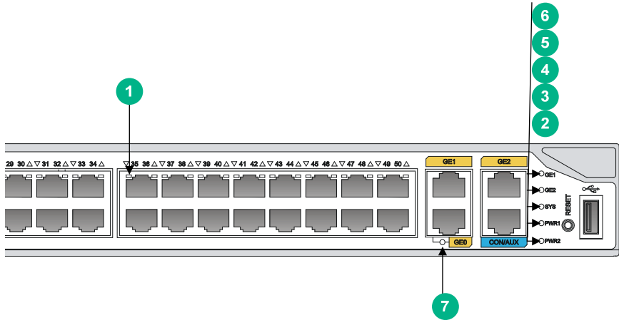
图B-2 R3900-S51 指示灯
