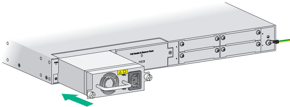
图2-17 R3900-S51 安装交流电源模块
