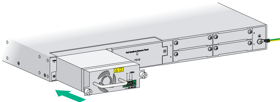
图2-18 R3900-S51 安装直流电源模块
