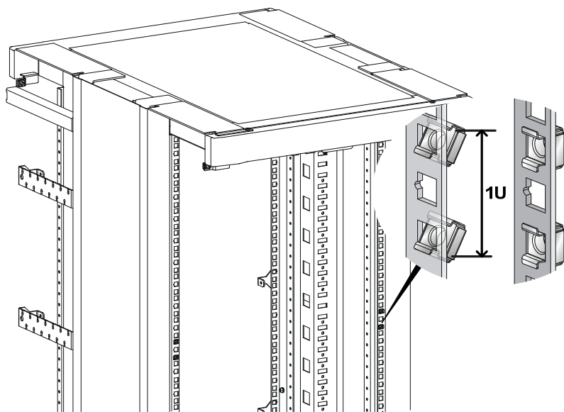
图2-8 安装浮动螺母
