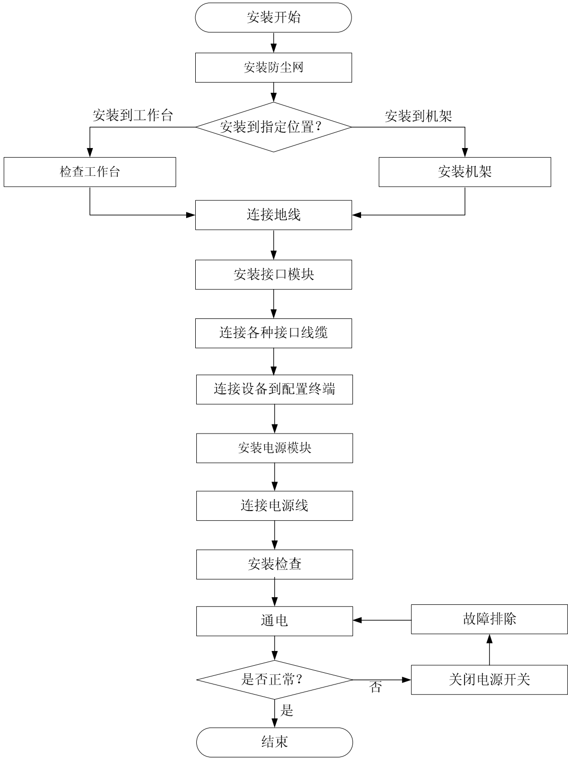
图2-1 设备安装流程图
