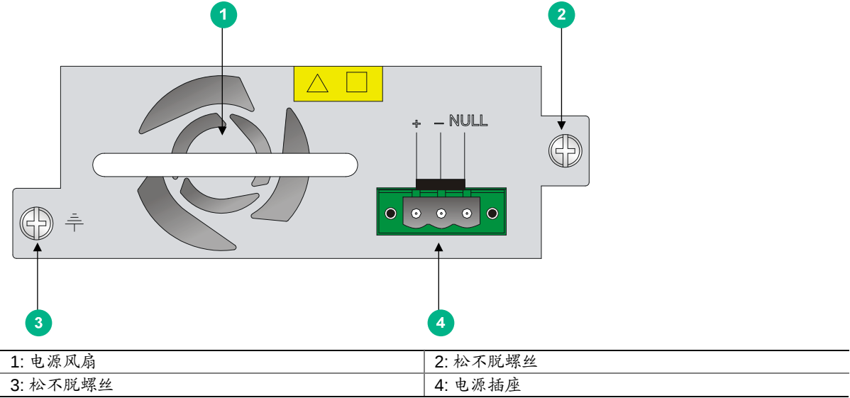
图A-6 R3900-S51 直流电源模块
