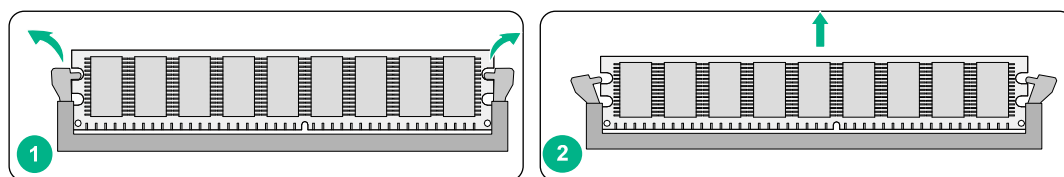
图3-2 拆卸内存
