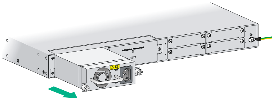
图3-1 将电源模块拉出电源插槽
