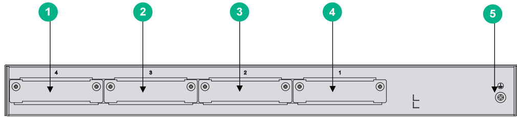
图A-2 R3900-S28 后视图
