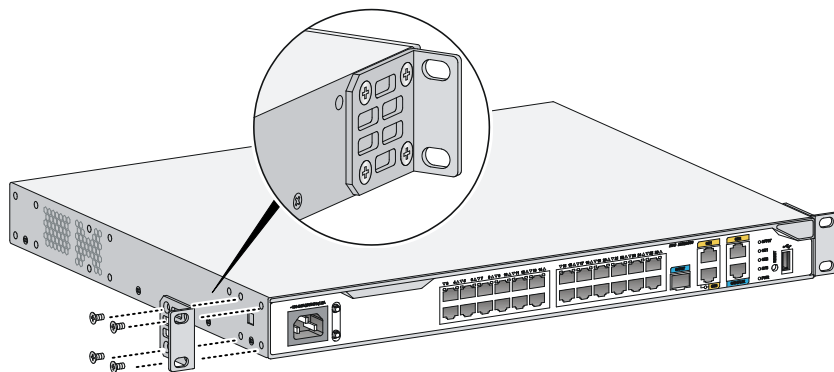
图2-9 安装挂耳到设备
